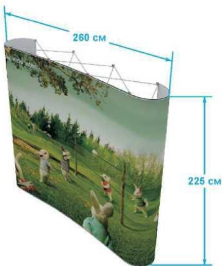
стандартная конструкция 3x3 секции
