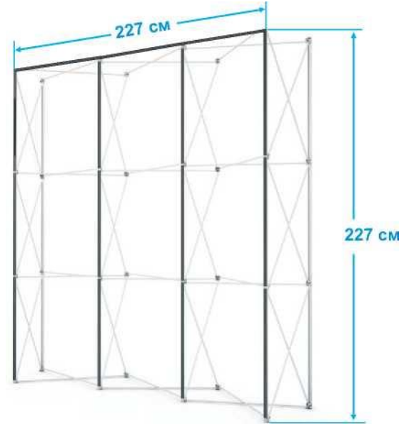
конструкция MEDUSA lite 3x3 секции рекламное полотно - банер
